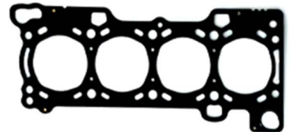
1,10mm 1 Agujero Junta de culata OEM N.º: 500387067 Avortex N.º: 605
