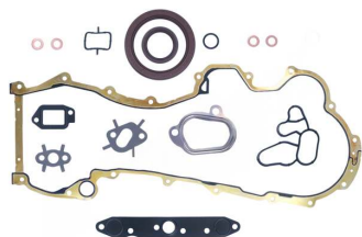
Juego de juntas inferior OEM N.º: 71744286 Avortex N.º: 230
