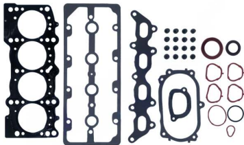
Juego de juntas de culata OEM N.º: 71716870 Avortex N.º: 285
