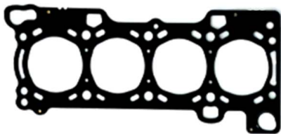
1,20mm 2 Agujero Junta de culata OEM N.º: 500387068 Avortex N.º: 606
