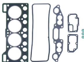
Juego de juntas de culata OEM N.º: 7701458694U Avortex N.º: 543
