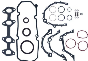
Juego completo de juntas sin junta de culata OEM N.º: 71740655F Avortex N.º: 2950S
