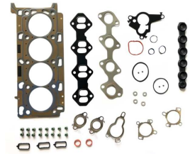
Juego de juntas de culata OEM N.º: 7701479334 Avortex N.º: 741
