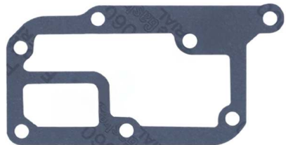
Junta de bomba de agua R-9 (pequeño - con oreje... OEM N.º: N/A Avortex N.º: 1821511
