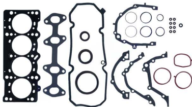
Juego completo de juntas OEM N.º: 71740655F Avortex N.º: 295
