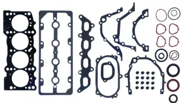
Juego completo de juntas OEM N.º: 71716871 Avortex N.º: 280
