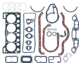
Juego de juntas de motor completo OEM N.º: 7701458694 Avortex N.º: 540
