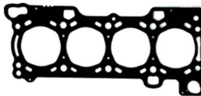
1,30mm 3 Agujero Junta de culata OEM N.º: 500387069 Avortex N.º: 607
