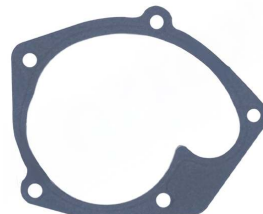
Junta de bomba de agua OEM N.º: 7700115278 Avortex N.º: 412
