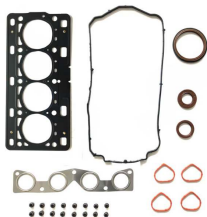
Juego completo de juntas OEM N.º: 7701475822 Avortex N.º: 459
