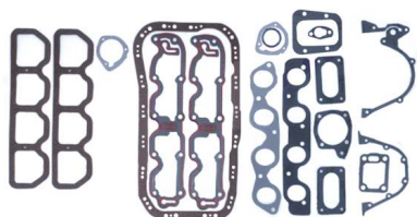
Juego de juntas de motor sin junta de culata OEM N.º: 5893326 Avortex N.º: 3610S
