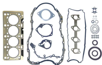
Juego completo de juntas OEM N.º: 7701477501F Avortex N.º: 710
