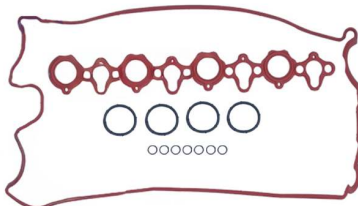
Junta de tapa de válvulas Juego OEM N.º: 7701472450 Avortex N.º: 483
