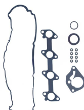
Juego de juntas de culata sin junta de culata OEM N.º: 7701473371 Avortex N.º: 4020S
