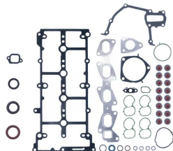
Juego completo de juntas sin junta de culata OEM N.º: 71769851S Avortex N.º: 381
