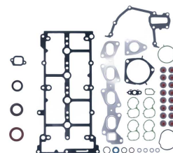
Juego completo de juntas sin junta de culata OEM N.º: 71769851CF Avortex N.º: 383
