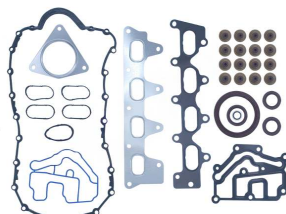
Juego completo de juntas sin junta de culata OEM N.º: 7701471886F Avortex N.º: 4200S
