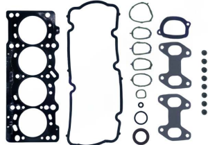
Juego de juntas de culata OEM N.º: 71718503 Avortex N.º: 260
