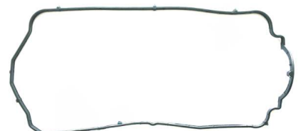
Junta de tapa de válvulas OEM N.º: 7701059314 Avortex N.º: 455
