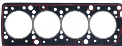
Junta de culata OEM N.º: 7709257 Avortex N.º: 362
