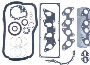
Juego completo de juntas sin junta de culata OEM N.º: 7701468142F Avortex N.º: 4600S
