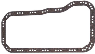
Junta de cárter de aceite OEM N.º: 7554363 Avortex N.º: 2632110
