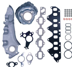
Juego de juntas de culata sin junta de culata OEM N.º: 101015474R Avortex N.º: 8010S
