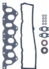
Juego de juntas de culata sin junta de culata OEM N.º: 7701463110 Avortex N.º: 5260S
