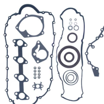
Juego completo de juntas sin junta de culata (Cort... OEM N.º: 7701473371C Avortex N.º: 4030S
