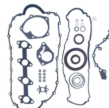
Juego completo de juntas sin junta de culata OEM N.º: 7701473371S Avortex N.º: 505
