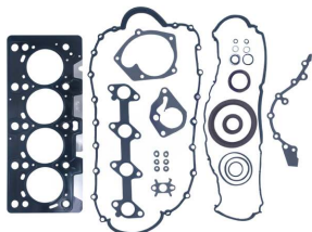
Juego completo de juntas (Sello de aceite de Viton... OEM N.º: 7701473371F Avortex N.º: 401
