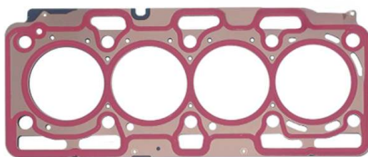
Junta de culata OEM N.º: 110447055R Avortex N.º: 703
