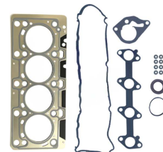
Juego de juntas de culata OEM N.º: 7701476729 Avortex N.º: 416
