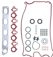
Juego de juntas de culata sin junta de culata OEM N.º: 7701475278 Avortex N.º: 4810S
