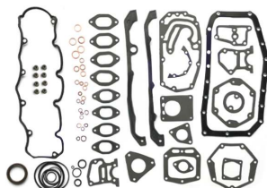
Juego completo de juntas sin junta de culata OEM N.º: 7701206361F Avortex N.º: 4700S
