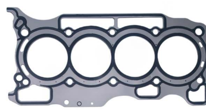
Junta de culata OEM N.º: 110445H60A Avortex N.º: 722
