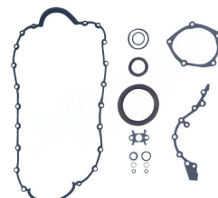
Комплект нижних прокладок двигателя OEM №: 7701473371A Avortex №: 414
