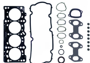
Комплект прокладок головки блока цилиндров OEM №: 71718503 Avortex №: 260
