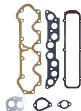
Комплект прокладок ГБЦ без прокладки ГБЦ OEM №: 71737120H Avortex №: 3390S
