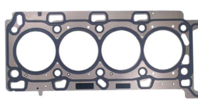
Прокладка головки блока цилиндров OEM №: 110448588R Avortex №: 732
