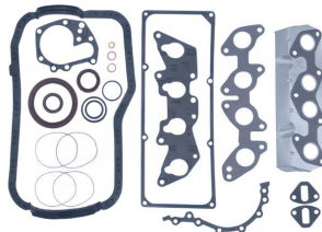
Полный комплект прокладок без прокладки ГБЦ OEM №: 7701468142F Avortex №: 4600S
