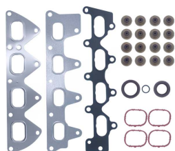
Комплект прокладок ГБЦ без прокладки ГБЦ OEM №: 7701474372 Avortex №: 5910S
