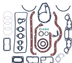
Полный комплект прокладок без прокладки ГБЦ OEM №: 7701460627 Avortex №: 5410S
