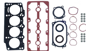
Комплект прокладок головки блока цилиндров OEM №: 71749165 Avortex №: 651
