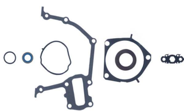
Комплект нижних прокладок двигателя OEM №: 71749743 Avortex №: 385
