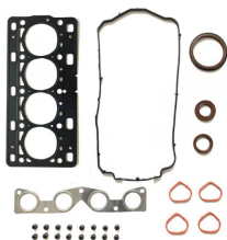
Полный комплект прокладок OEM №: 7701475822 Avortex №: 459
