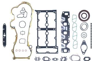
Полный комплект прокладок без прокладки ГБЦ OEM №: 71744285 Avortex №: 235
