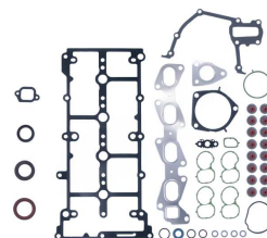
Полный комплект прокладок без прокладки ГБЦ OEM №: 71769851CF Avortex №: 383
