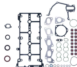
Полный комплект прокладок без прокладки ГБЦ OEM №: 71769851CF Avortex №: 383
