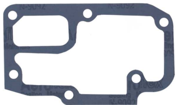
R-12 Прокладка водяного насоса (малый - Pencereci) OEM №: N/A Avortex №: 1821211
