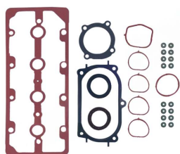
Комплект прокладок ГБЦ без прокладки ГБЦ OEM №: 71749165 Avortex №: 6510S
