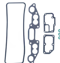
Комплект прокладок ГБЦ без прокладки ГБЦ OEM №: 7701458694U Avortex №: 5430S
