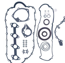
Полный комплект прокладок без прокладки ГБЦ OEM №: 7701473371S Avortex №: 505
