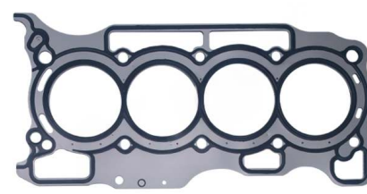
Прокладка головки блока цилиндров OEM №: 110445H60A Avortex №: 722
