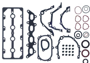
Полный комплект прокладок без прокладки ГБЦ OEM №: 71716871 Avortex №: 2800S
