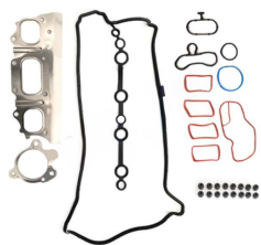
Комплект прокладок ГБЦ без прокладки ГБЦ OEM №: 101015303R Avortex №: 7510S
