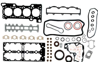
Полный комплект прокладок OEM №: 504049360F Avortex №: 602
