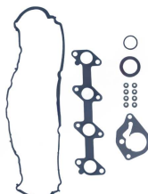
Комплект прокладок ГБЦ без прокладки ГБЦ OEM №: 7701473371 Avortex №: 4020S
