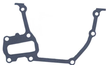
Прокладка масляного насоса OEM №: 71736256 Avortex №: 397
