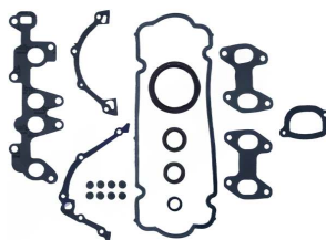
Полный комплект прокладок без прокладки ГБЦ OEM №: 71737117 Avortex №: 3100S
