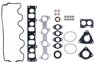
Комплект прокладок ГБЦ без прокладки ГБЦ OEM №: 71718658 Avortex №: 2210S
