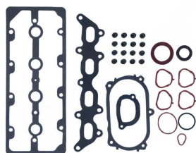
Комплект прокладок ГБЦ без прокладки ГБЦ OEM №: 71716870 Avortex №: 2850S
