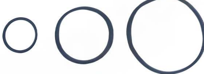
Комплект резиновых прокладок масляного фильтра OEM №: 7701473629 Avortex №: 418
