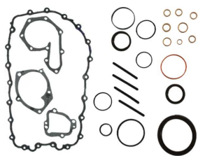
Комплект нижних прокладок двигателя OEM №: 7701466408 Avortex №: 495
