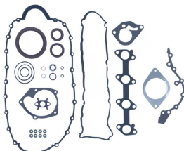
Полный комплект прокладок без прокладки ГБЦ OEM №: 7701476729F Avortex №: 4150S
