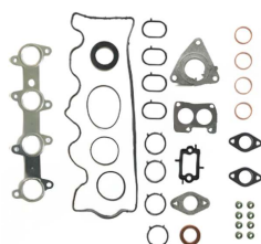
Комплект прокладок ГБЦ без прокладки ГБЦ OEM №: 71715699 Avortex №: 2410S
