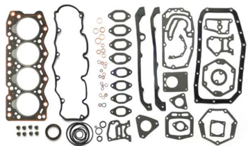
Полный комплект прокладок OEM №: 71728336F Avortex №: 610
