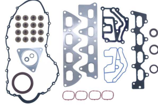
Full Takım Conta SKC Hariç OEM No: 7701474372F Avortex No: 5900S
