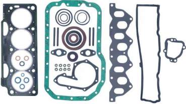
Full Takım Conta OEM No: 7701466406 Avortex No: 520
