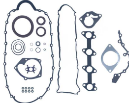
Full Takım Conta SKC Hariç OEM No: 7701476729F Avortex No: 4150S
