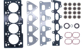
Üst Takım Conta OEM No: 7701474372 Avortex No: 591
